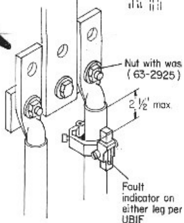
DOUBLE LUG ASSEMBLY
